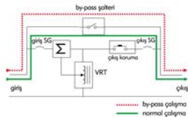
ERG-ESV-1XX/1 FAZ SERVO OTOMATİK REGÜLATÖR SİSTEMİ
