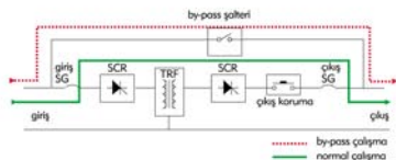
IMPACT 1XX 1 FAZ STATİK REGÜLATÖR SİSTEMİ
